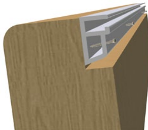
Figure 29 – Pose du rail d'accrochage
