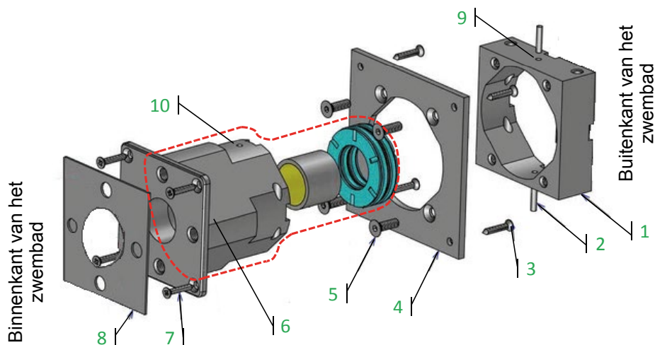
Figuur 25 – Plaatsing van de wanddoorvoer
