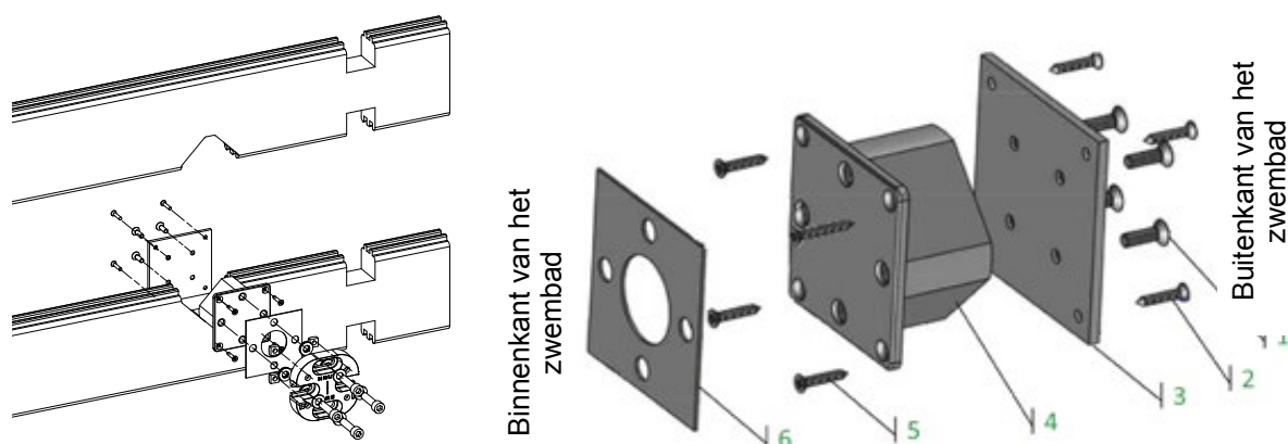
Figuur 27 – Montage van de steunlager
