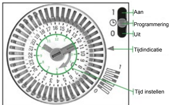
Figuur 57 – Voorzijde van de filterklok
