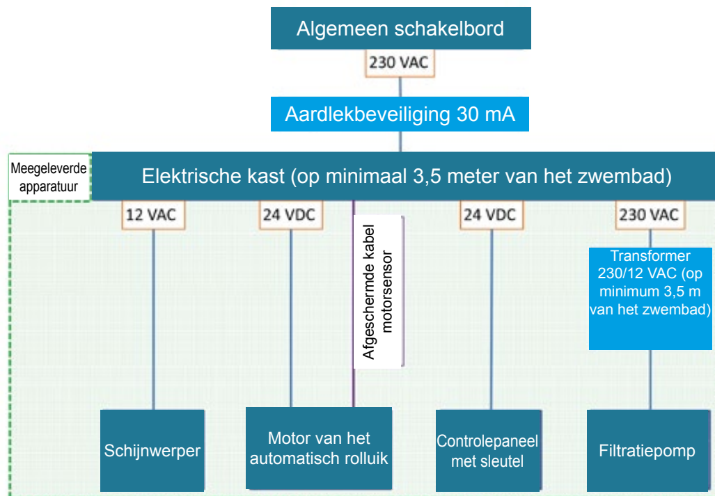
Figuur 54 – Elektrisch blokschema van het STADSZWEMBAD
