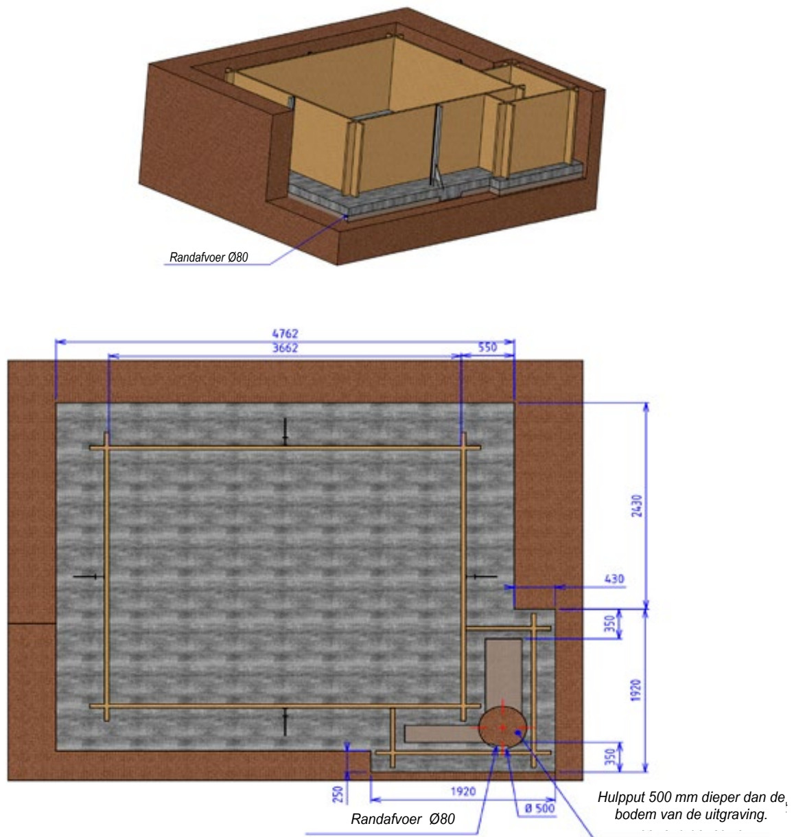
Figuur 1 – Montage van het drainagesysteem
