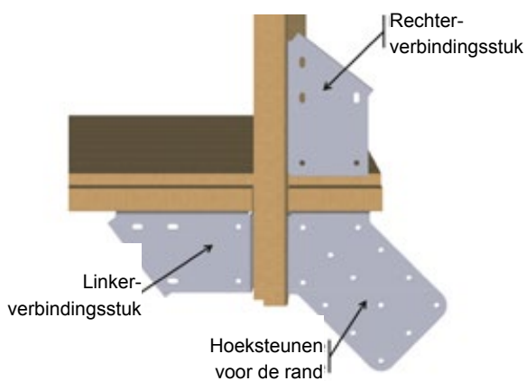
Figuur 18 – Het plaatsen van de verbindingstukken in de hoeken
