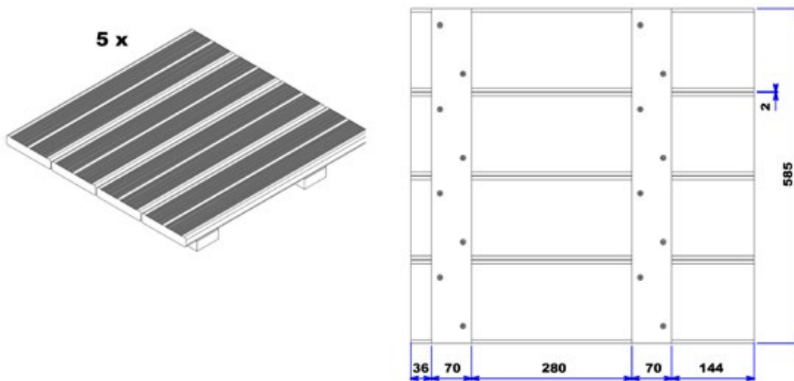
Figuur 51 – Montage van de vlonders
