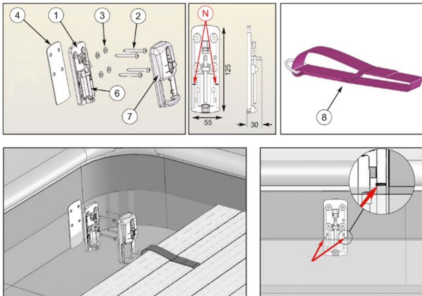
Figuur 46 – De bevestigingsbanden van de afdekking plaatsen
