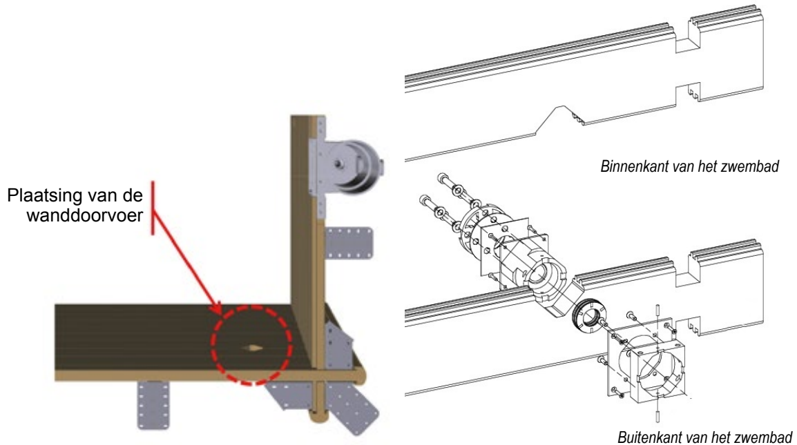
Figuur 25 – Plaatsing van de wanddoorvoer
