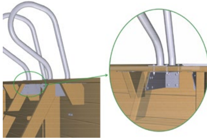
Figuur 53 – De handgrepen van de ladder vastzetten
