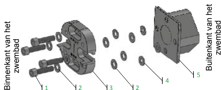
Figuur 36 – Montage van de flens van de lagersteun
