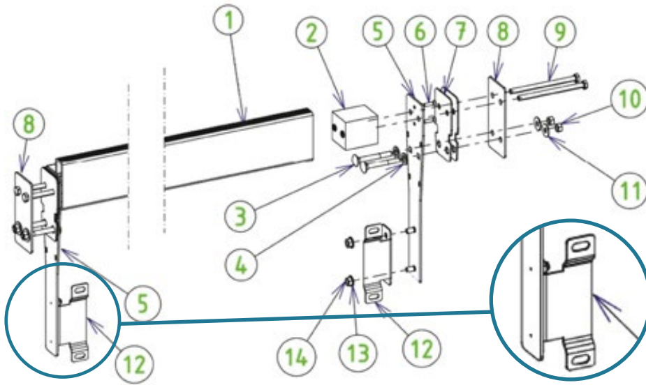
Figuur 41 – Montage en installatie van de steunbalk
