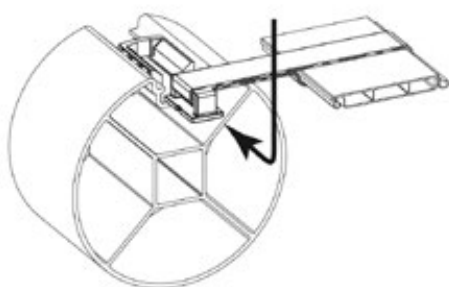
Figuur 45 – Verbinding van de afdekking met de as
