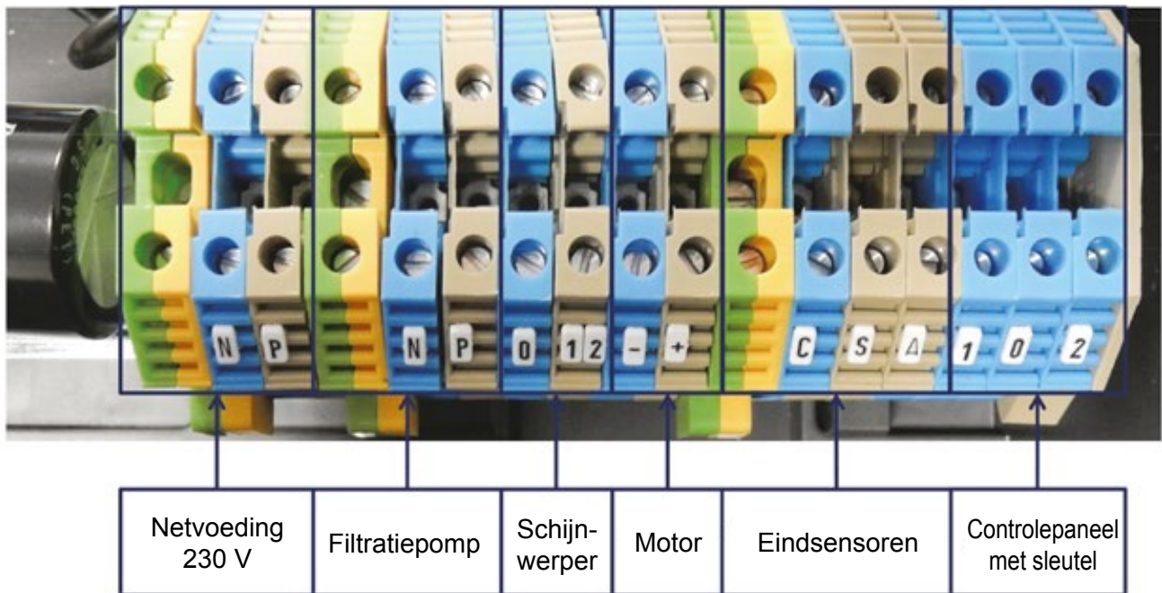
Figuur 55 – Schakelkast voor het STADSZWEMBAD
