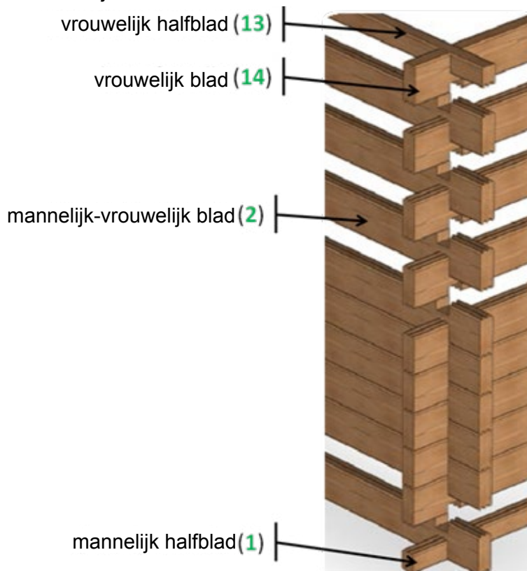
Figuur 9 – Principe van in elkaar grijpende houten latten
