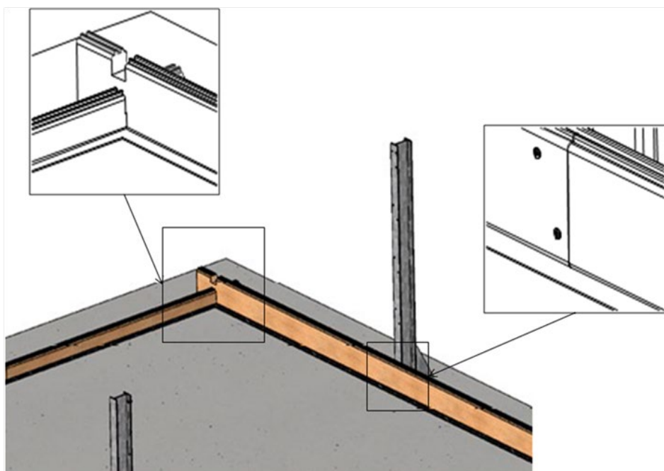
Figuur 10 – Onderlinge vergrendeling van de planken
