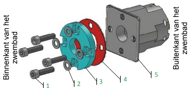
Figuur 35 – Montage van de flens voor de wanddoorvoer
