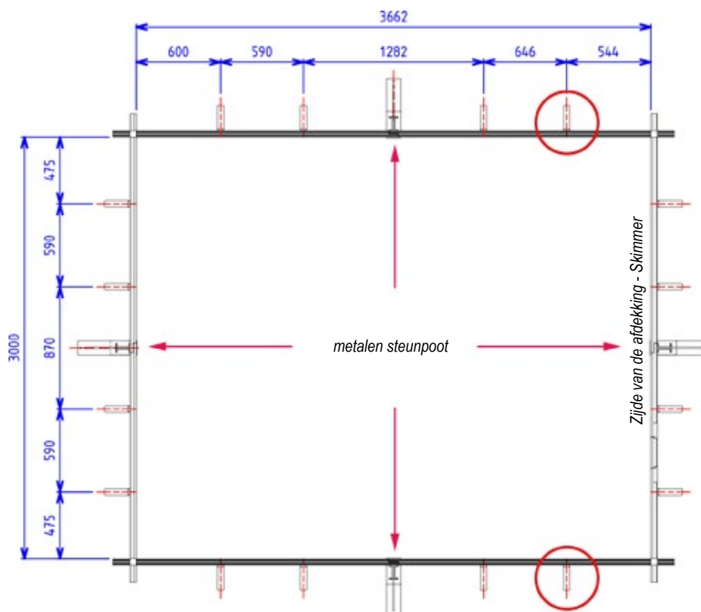
Figuur 14 – Locatie van de boordplanken
