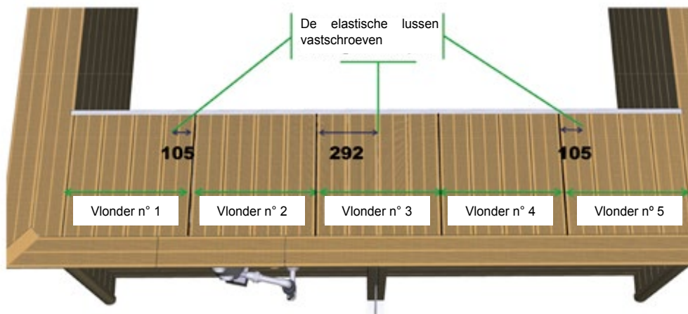
Figuur 52 – Bevestiging van elastische banden onder de vlonders
