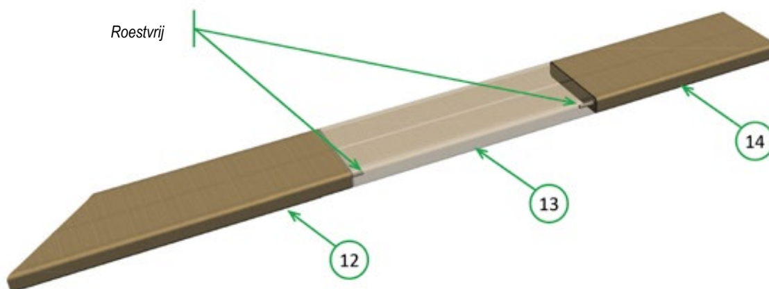
Figuur 49 – Montage van de scharnieren
