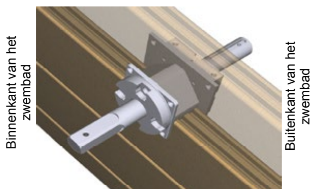
Figuur 38 – Montage van de as van het automatisch rolluik
